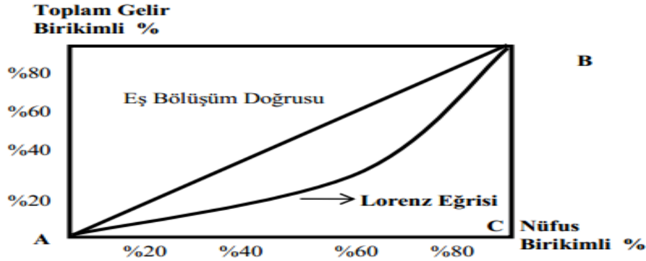
Şekil 1: Lorenz Eğrisi
